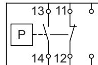
Schaltbild Druckschalter PMS-10 wiring diagram for pressure switch PMS-10
